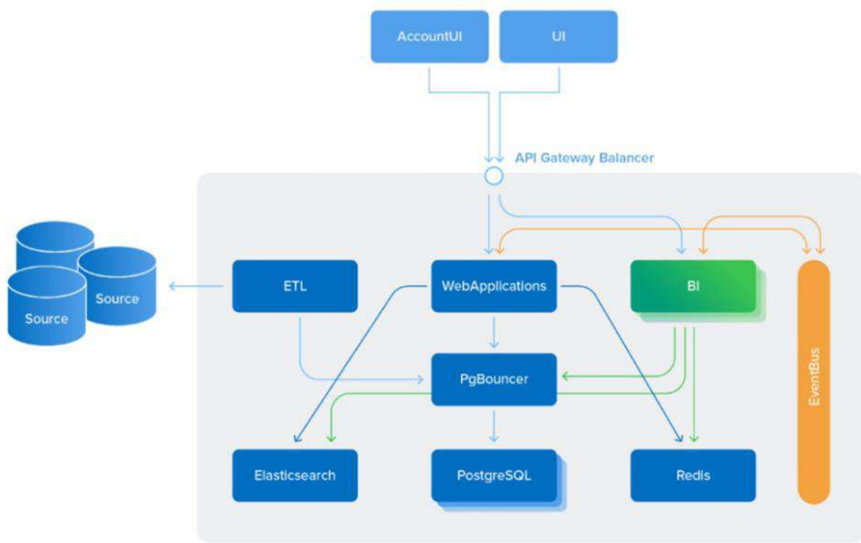
Рисунок 2 – Типовая архитектура веб-прилоеежня
